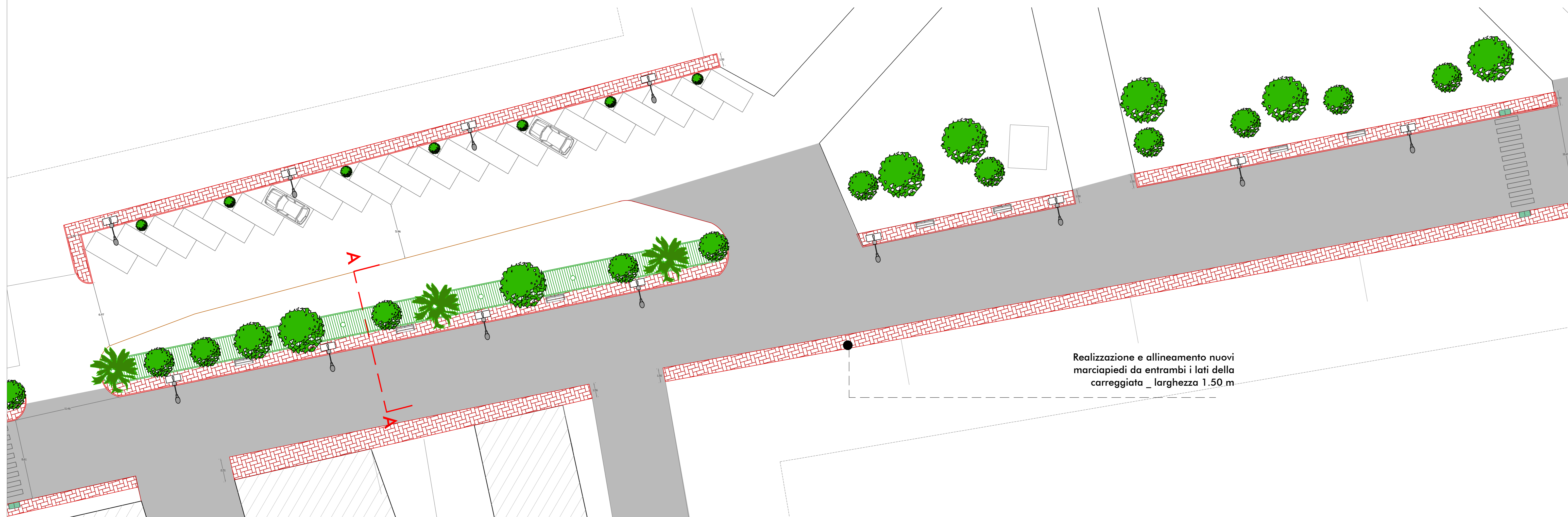
Stato di progetto_ planimetria TRATTO 2_ scala 1:200
